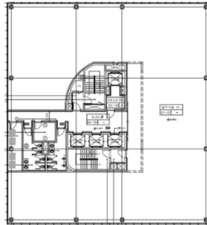
기준층 평면도
