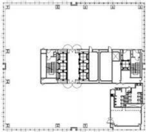
기준층 평면도
