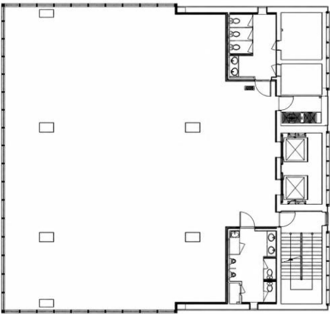
기준층 평면도
