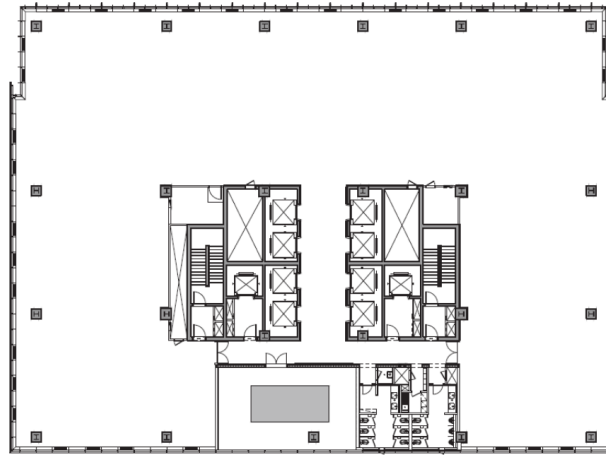
기준층 평면도
