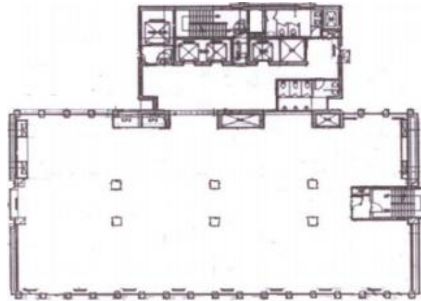
기준층 평면도
