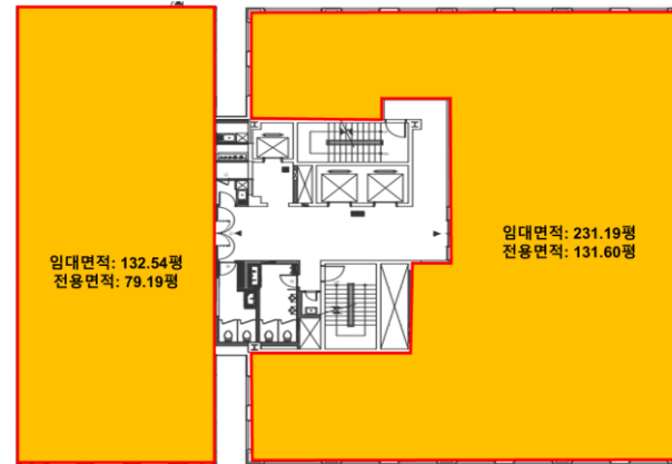
기준층 평면도
