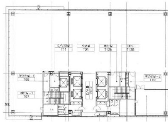
기준층 평면도
