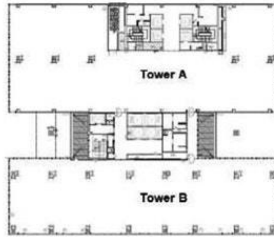
기준층 평면도
